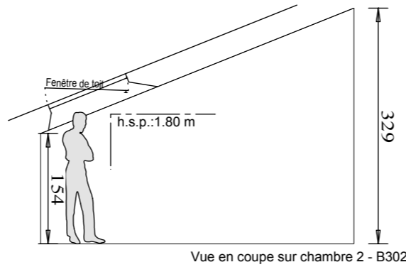
Vue en coupe sur chambre 2 - B302
